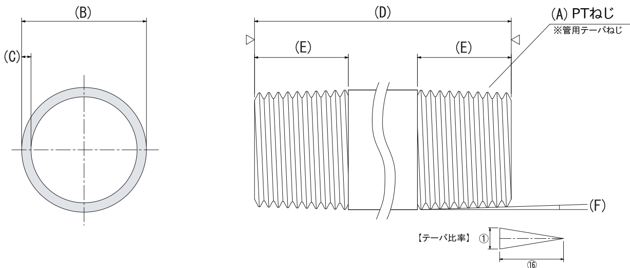
【ねじ詳細図】
