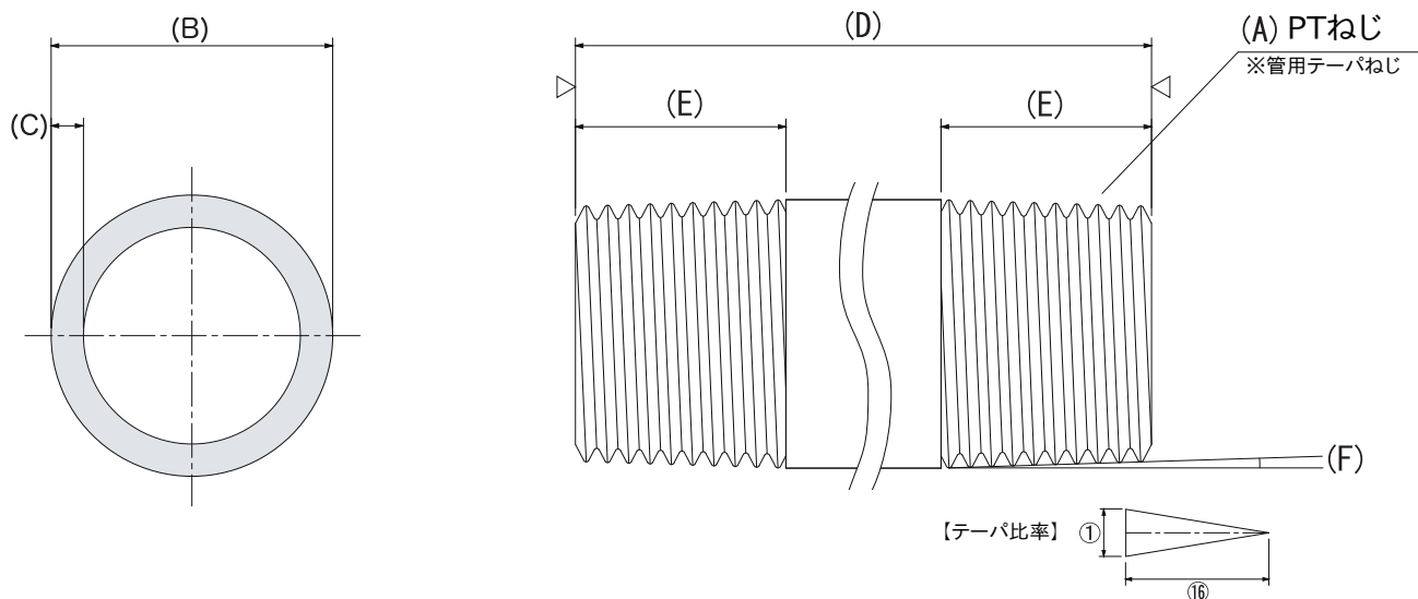
【ねじ詳細図】
