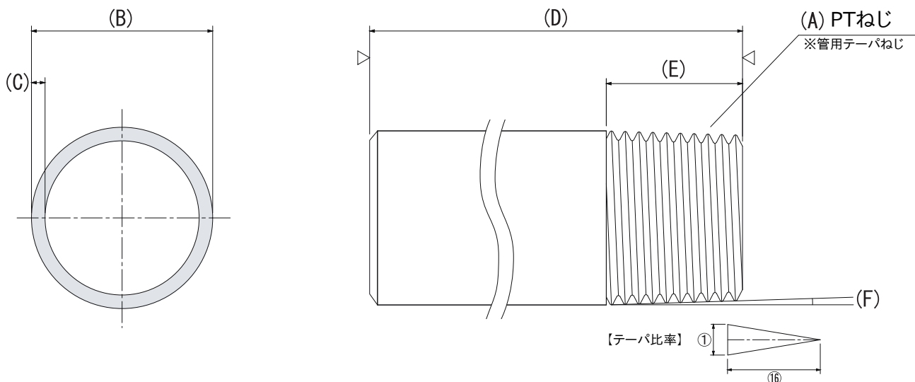
【ねじ詳細図】
